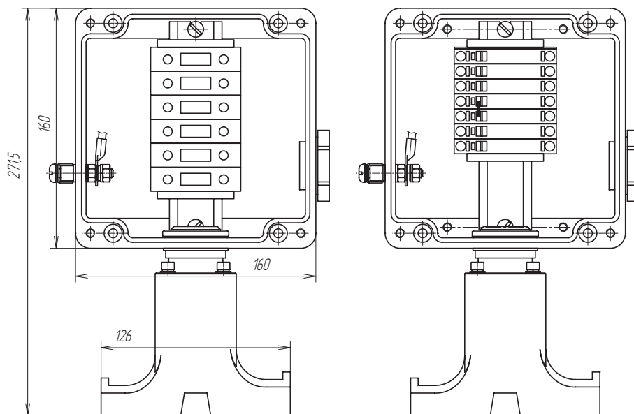
Коробка с винтовым клеммным блоком
